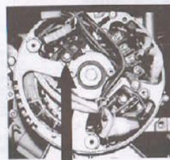
Figura D – Căutați locația perilor de cărbuni. Este posibil ca acest element să trebuiască să fie schimbat când se uzează excesiv.
